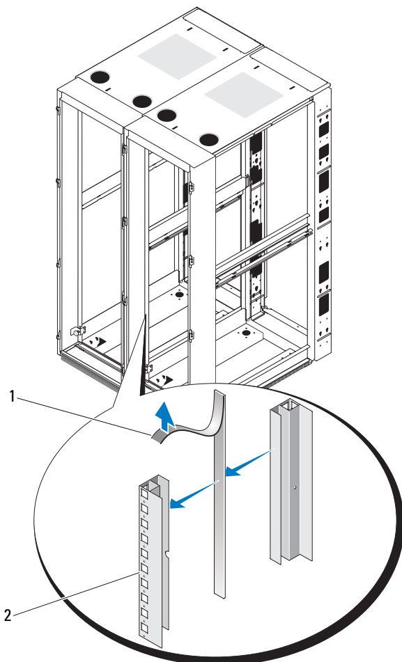
図 25. ガスケットテープの貼り付け
